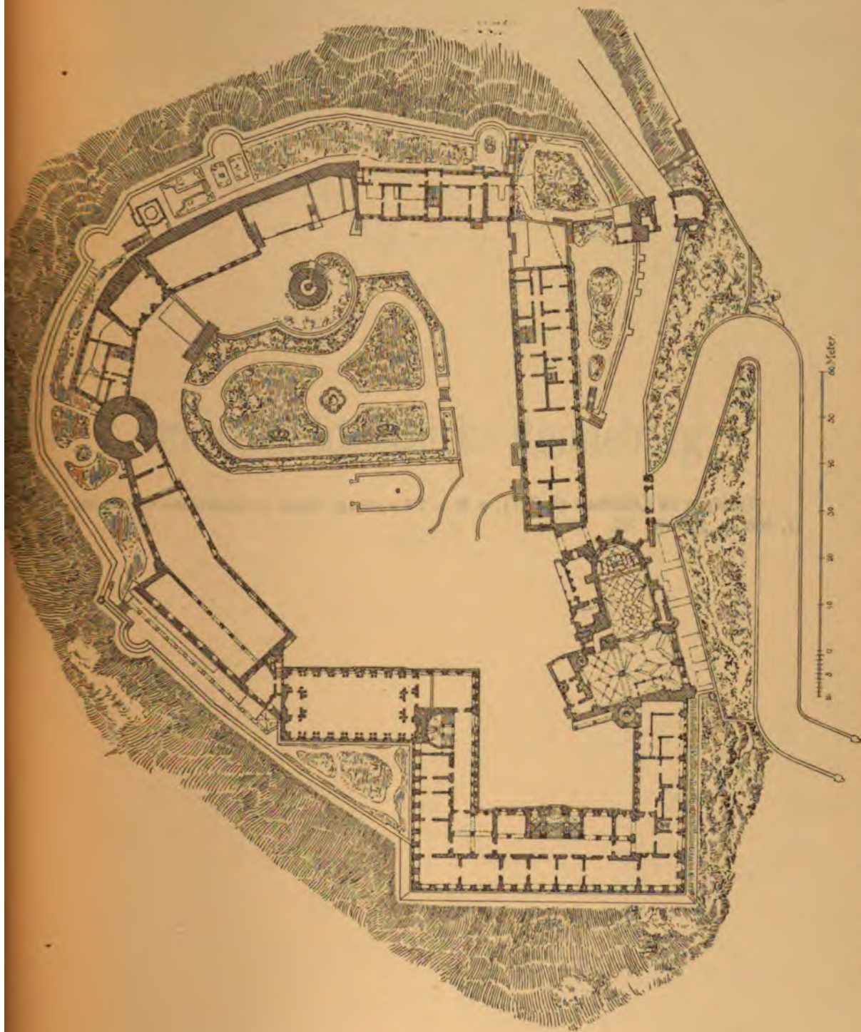
Grundriss des Schlosses Altenburg, neu aufgenommen für die Zwecke des Unternehmens, da der Grundriss auf S. 88 des Heftes Altenburg einige Bauten in ihrem Zustande vor 1868 wiedergab. Er ist dort irrthümlicher Weise als betreffs der neueren Bauten von Herrn Hofbaurath Kluge verbessert bezeichnet, was zu streichen ist.
